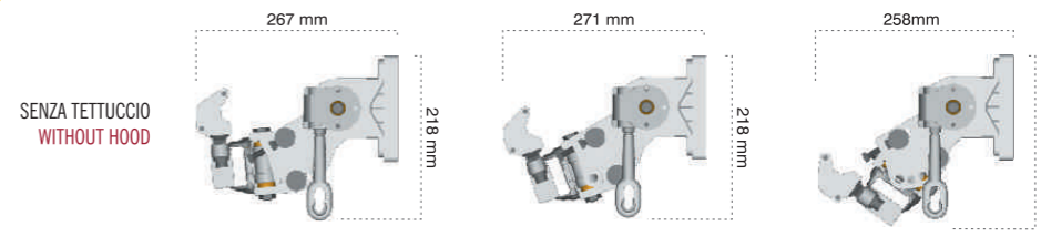
INGOMBRI / BULKS INCLINAZIONE / INCLINATION 5° INCLINAZIONE / INCLINATION 40° INCLINAZIONE / INCLINATION 70°
