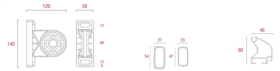
supporto universale universal fixing bracket profilo bracci "tipo L" "L" type arms profile profilo terminale terminal bar
